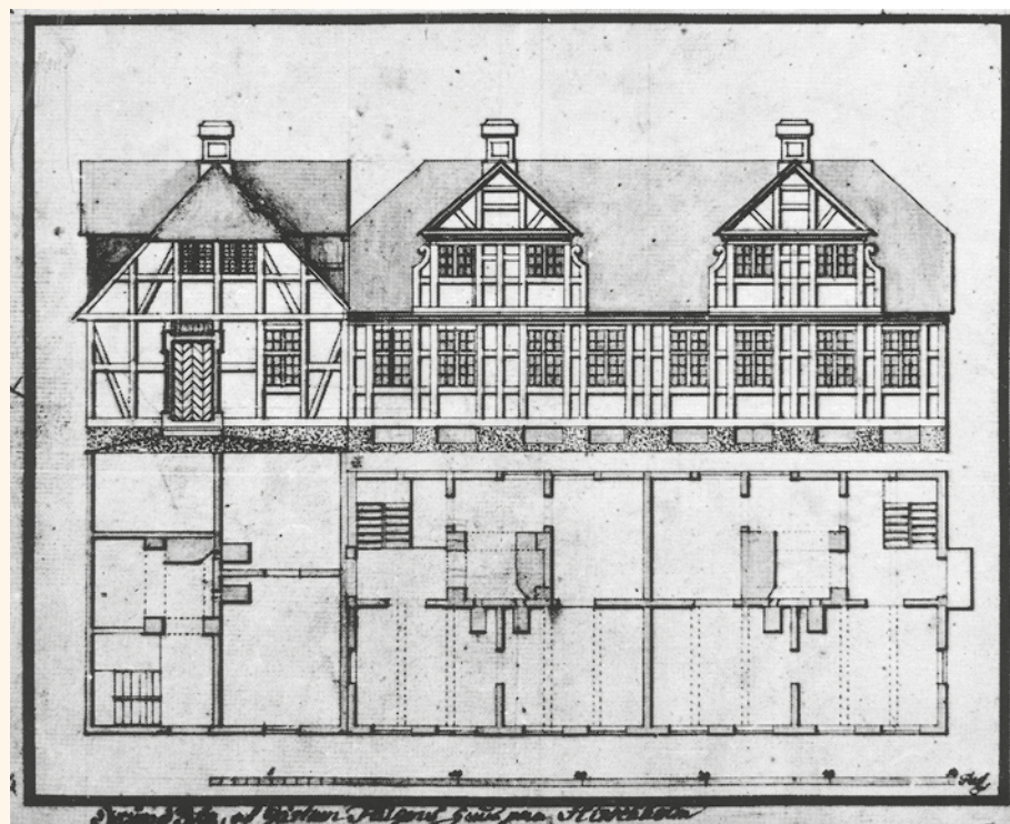
"Grundriss af Gartner Pflügers Huus på Hirschholm". Det er denne tegning, Pflügger indsendte til Hofmarskallen omkring 1760 med ansøgning om byggetilskud. Som beskrevet måtte Pflügger forenkle det endelige hus, og bl.a. stryge de store kviste. Originalen findes i Hofmarskallatets arkiv (Rigsarkivet), denne affotografering er i Hørsholms Lokalarkiv.
